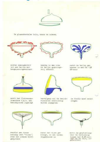
Montageschema voor zwart-wit beeldbuizen van Philips Stadskanaal, ca 1960 (bron: Philipsmuseum Stadskanaal)
